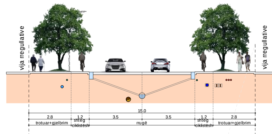
RRUGË PËRMBLEDHËSE 2-2
