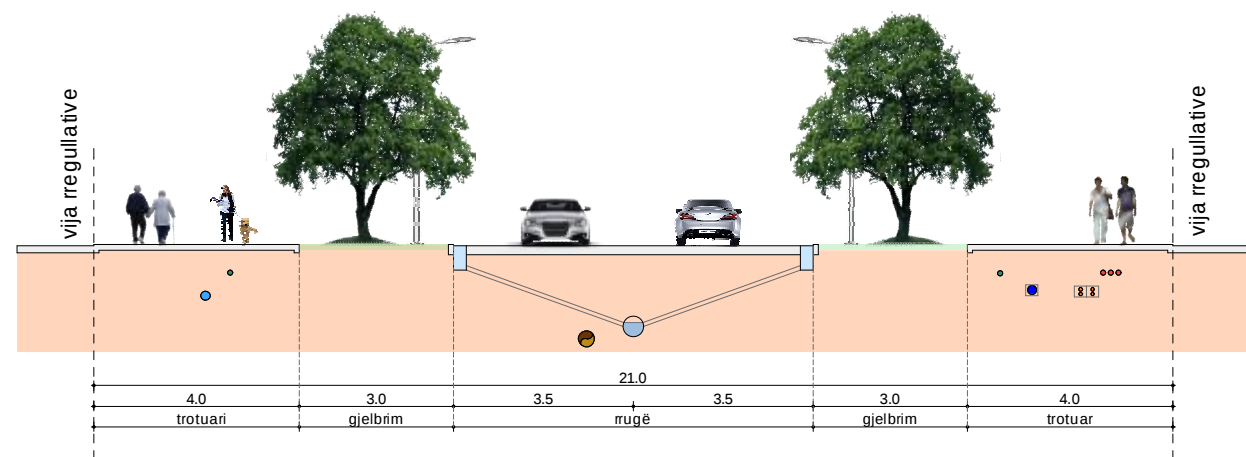
RRUGË PËRMBLEDHËSE 1-1
