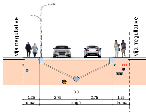
RRUGË LOKALE 4-4
