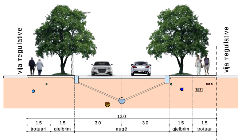
RRUGË PËRMBLEDHËSE 3-3
