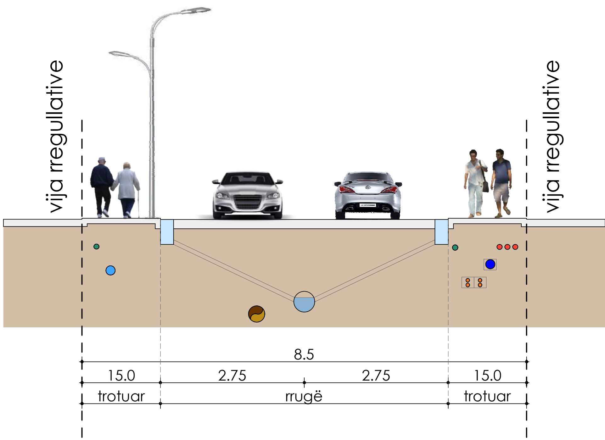
RRUGË LOKALE 4-4
