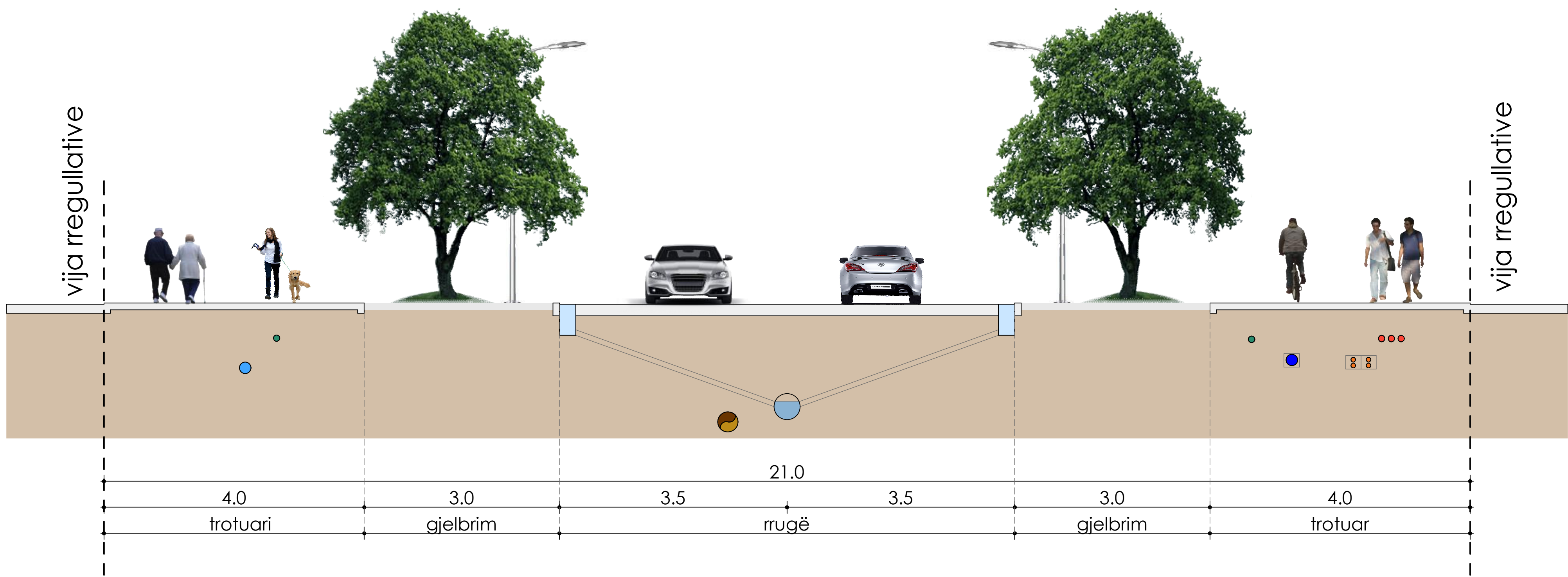
RRUGË PËRMBLEDHËSE 1-1
