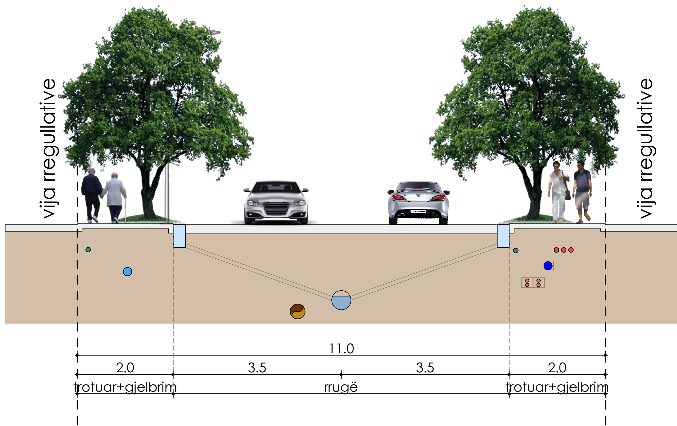
RRUGË PËRMBLEDHËSE 2-2
