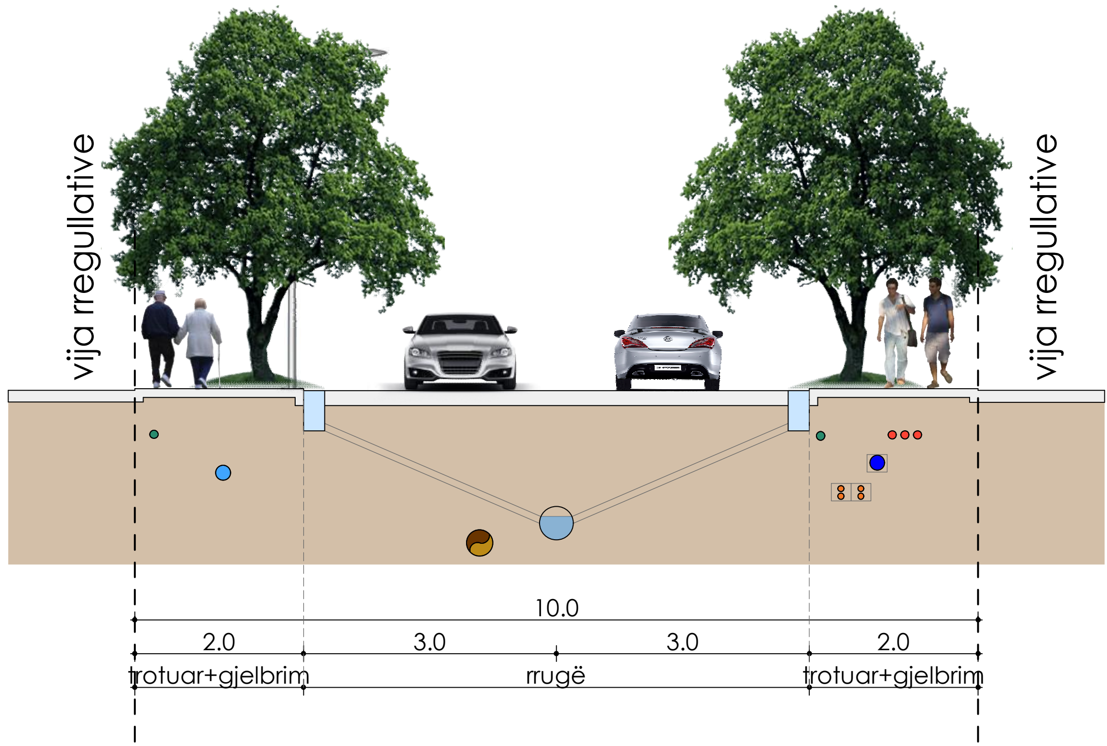
RRUGË PËRMBLEDHËSE 3-3
