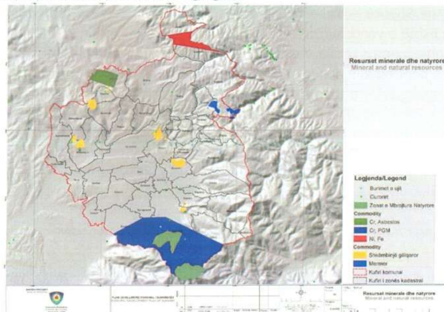
Figura 7 Resurset minerale
